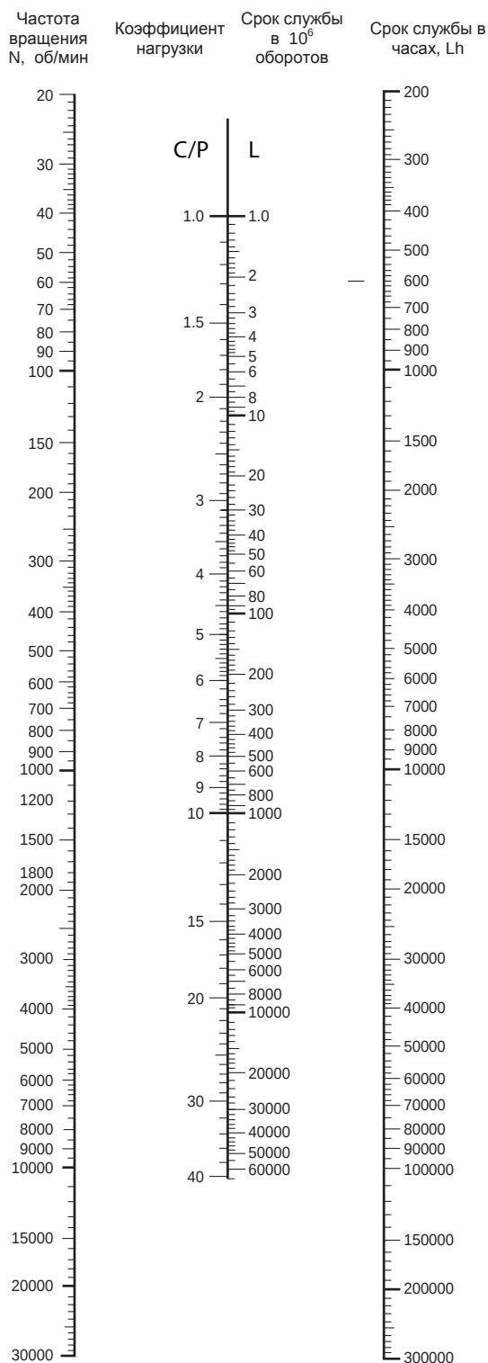
НОМОГРАММА (n-C/P-Lh)
